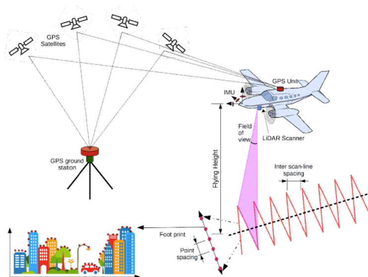
Figure 6 ALS Components 3
