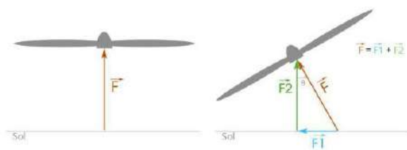
Figure 6 Portance et propulsion de l'hélice-(firediy.fr)
