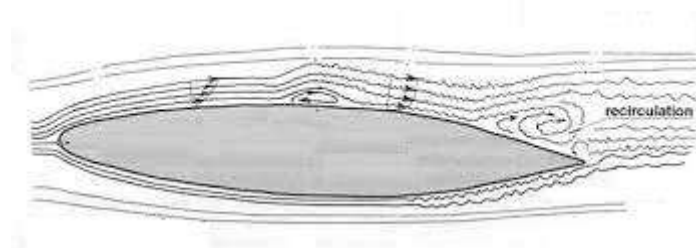
Figure 4 Filets d'air sur un profil
