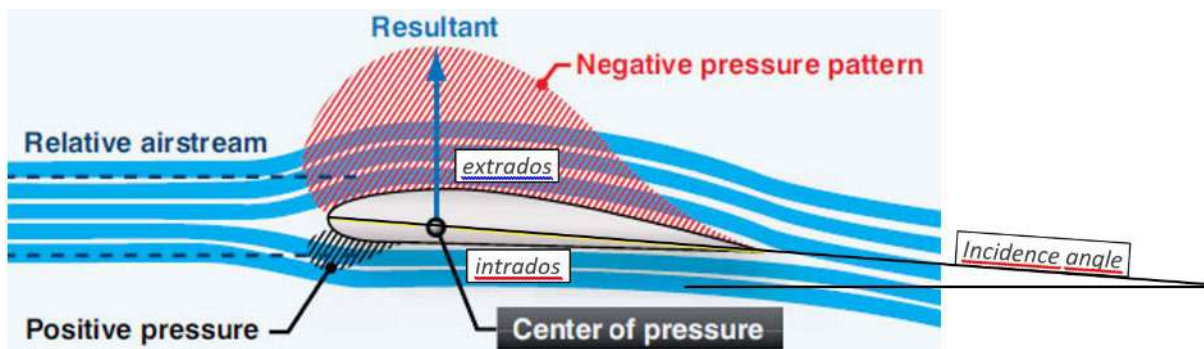
Figure 1 Portance de l'aile - (flight-mechanic.com-modifié)
