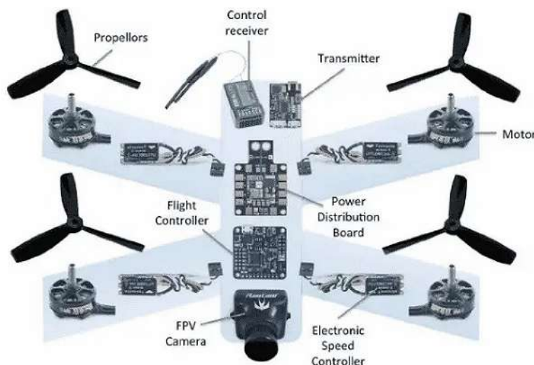
Figure 10 Composants électroniques du drone (10.wp.com)
