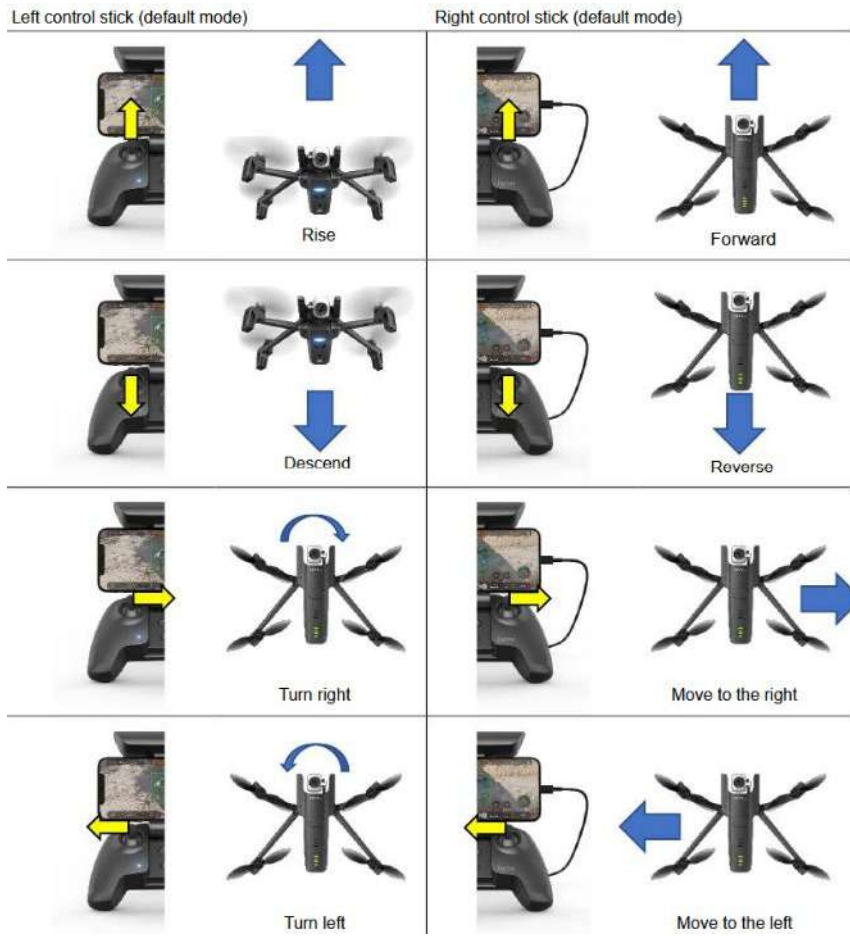
Figure 32 Contrôle du drone en mode 2 (manuel Parrot Anafi)
