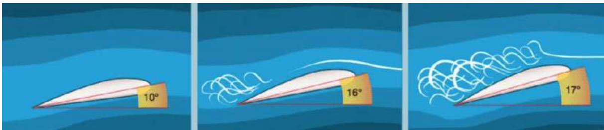
Figure 2 Décrochage (researchgate.net/profile/Mariateresa-Sestit)
