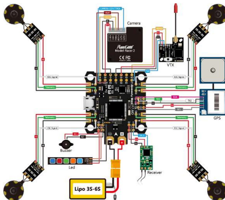
Figure 12 Liaisons vers le contrôleur de vol - phaserfpv.com.au
