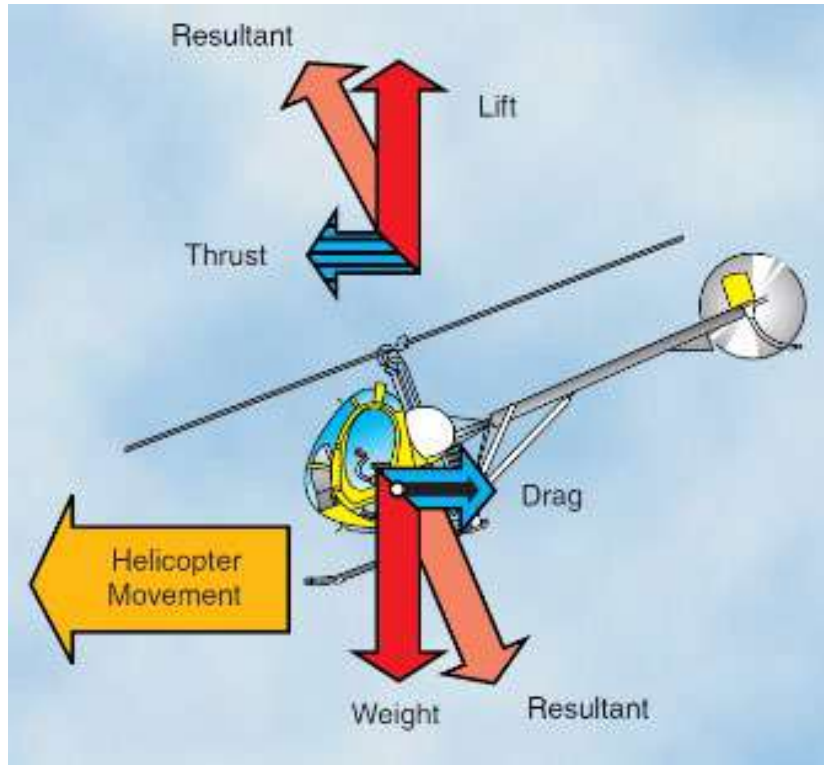
Figure 7 Un hélicoptère s'incline vers l'avant pour avancer-(aircraftsystemstech.com)
