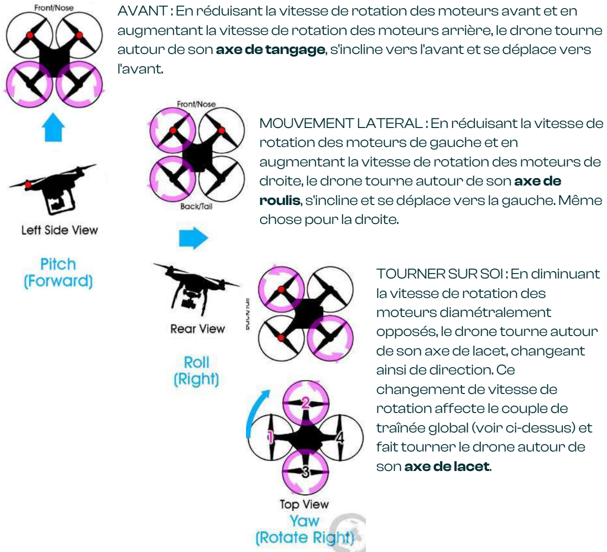
Figure 8 Actions des hélices pour diriger un drone multirotoeur (ipinimg.com)
