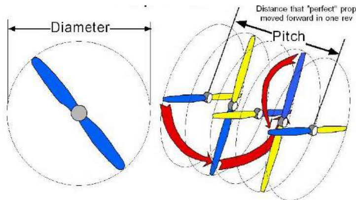
Figure 23 Définition de l'hélice (bowersflybaby.com)
