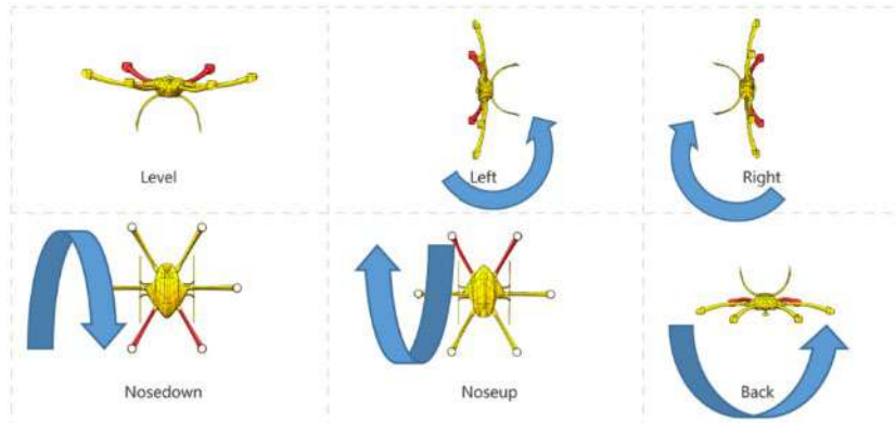
Figure 15 Mouvements d'étalonnage du magnétomètre autour de chaque axe - yangdaonline.com
