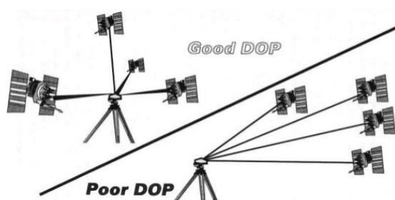
Figure 6-5 DOP depending on satellites position (KAnsari)
